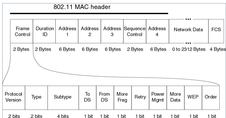
Rysunek 1. Format ramki IEEE 802.11 [22].
