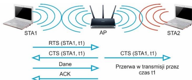
Rysunek 3. Działanie mechanizmu Request to Send/Clear to Send.
