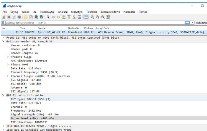
Rysunek 4. Ramka nawigacyjna interpretowana w programie Wireshark (informacje opisujące warstwę fizyczną).
