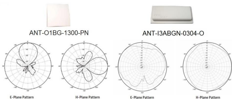
Rysunek 7. Rozkłady natężenia pola elektromagnetycznego przy częstotliwości 2,4 GHz dla zewnętrznej anteny kierunkowej ANT-O1BG-1300-PN o wzmocnieniu 13 dBi oraz anteny dookólnej ANT-I3ABGN-0304-O o wzmocnieniu 3 dBi.
