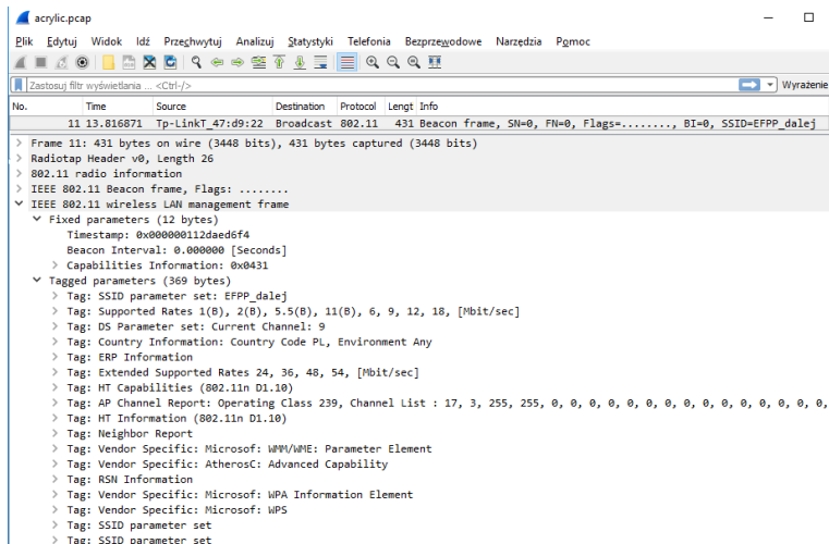
Rysunek 6. Ramka nawigacyjna interpretowana w programie Wireshark (informacje dotyczące rozgłaszanej sieci radiowej).
