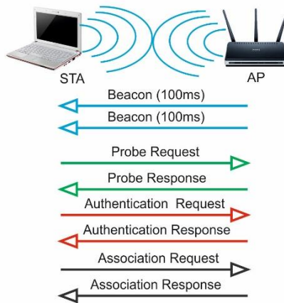
Rysunek 2. Etapy przyłączenia klienta do sieci bezprzewodowej.
